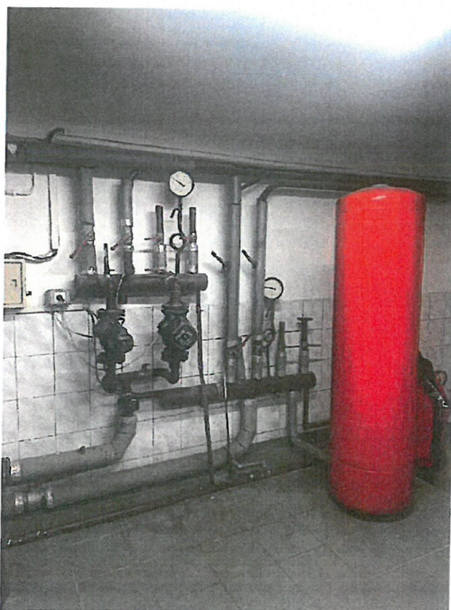
Zdjęcie 4 rozdzielacze oraz naczynie wzbiornicze przeponowe
